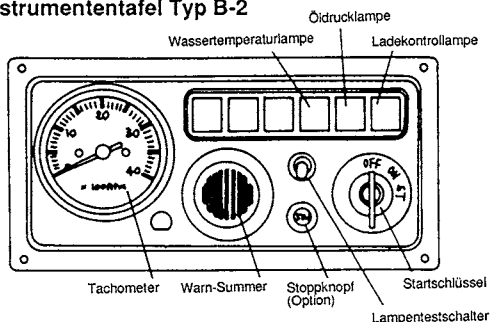
Instrumententafel Typ B-2
