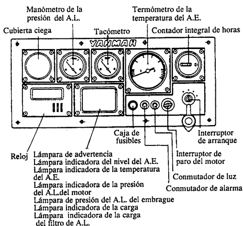
Panel de mando Tipo-D
