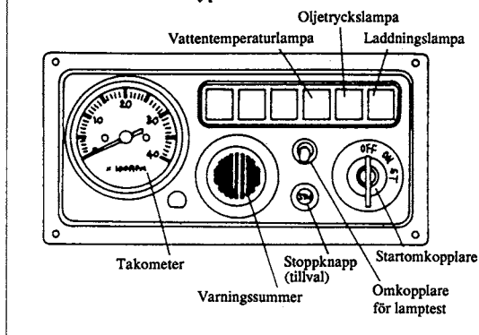
Instrumentbräde av typ B-2
