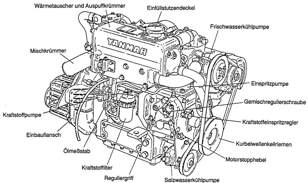
Auspuffseite 3GM30F
