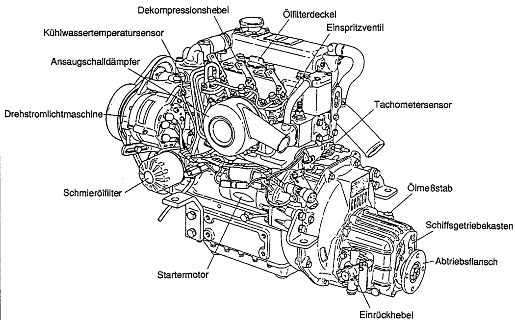
Ansaugseite 3GM30F
